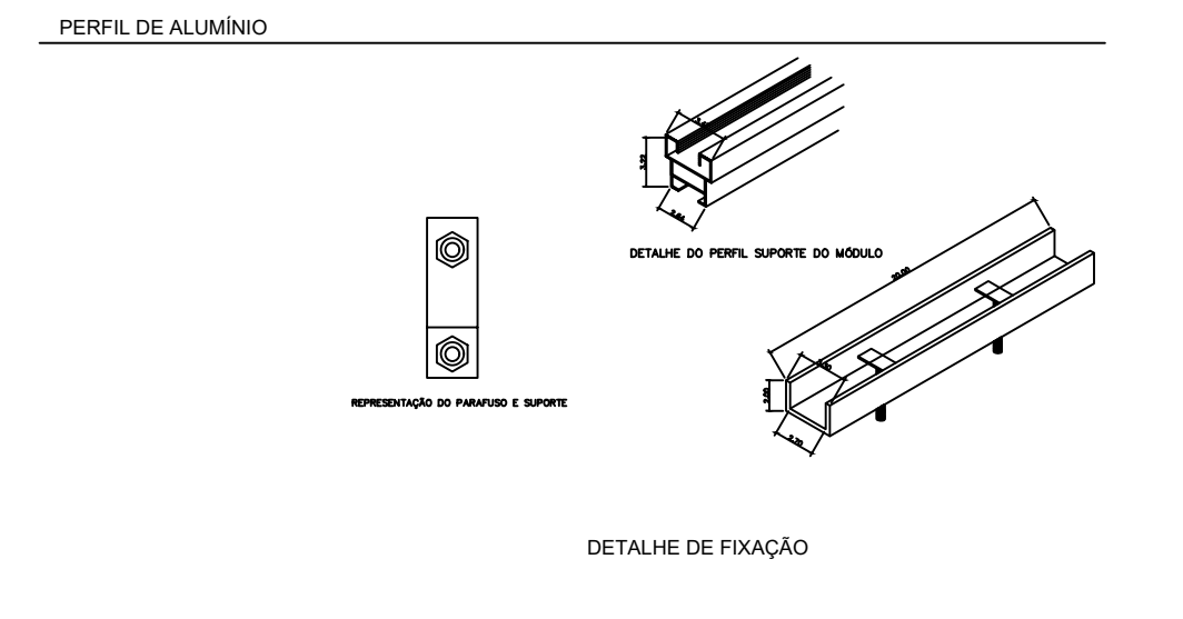
PERFIL DE ALUMÍNIO
