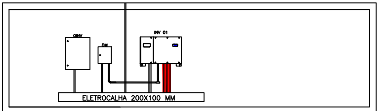
VISTA FRONTAL DOS INVERSORES E QUADROS
