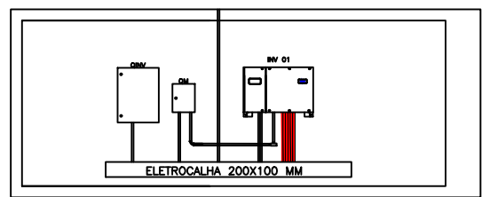
VISTA FRONTAL DOS INVERSORES E QUADROS
