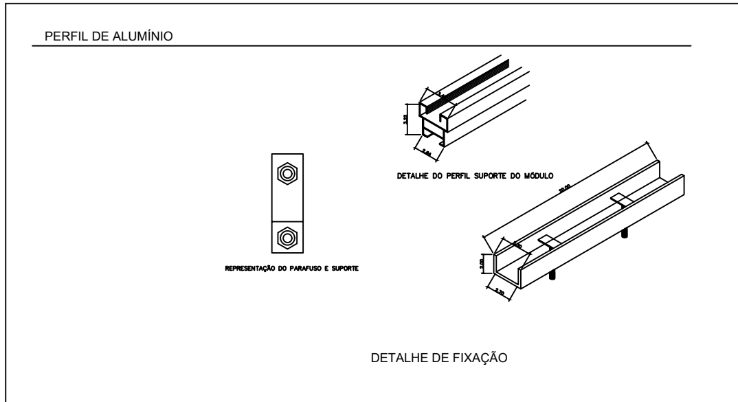
DETALHE DE FIXAÇÃO
